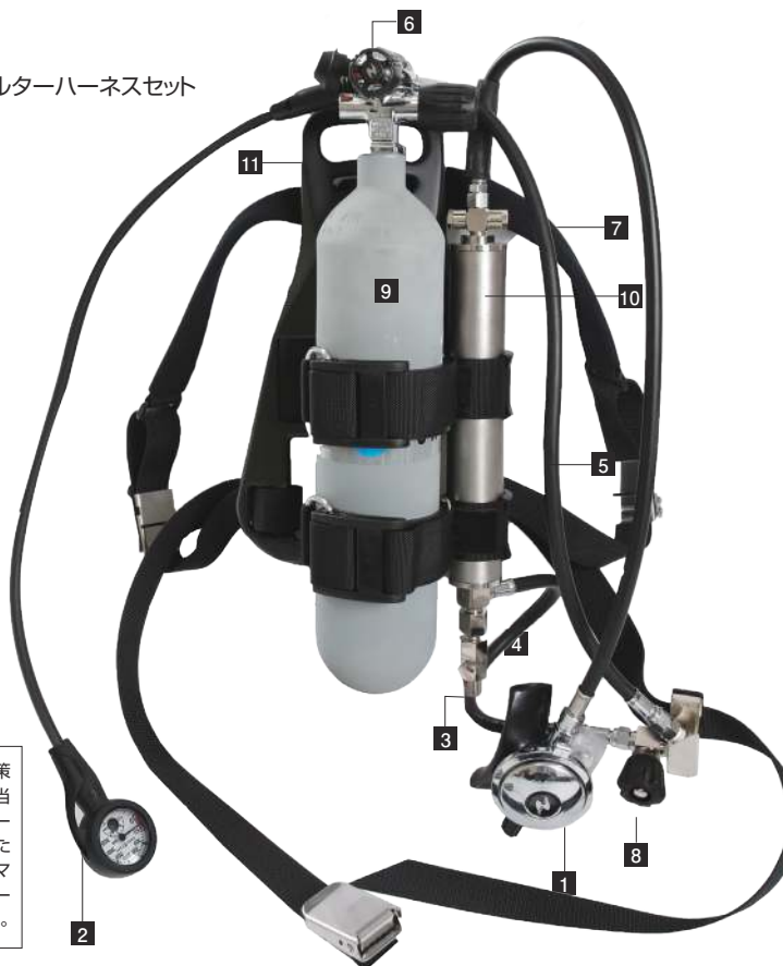
10 フィルター本体 税込価格 ¥33,000 ■タイプ:Nタイプ、Tタイプ ※LPプラグは付属されません。
