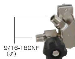
マニホールド ブロック 税込価格 ¥38,500 ※右脇腹付近に取り付け、フーカーホースとタンクのエア供給を切り換えることができます。
