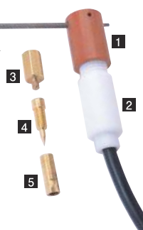
税込価格 ¥18,700 ※キャブタイヤなし ※溶接 (切断) 棒なし (パーツ) 1 キャップ部 税込価格 ¥9,680 2 グリップ部 税込価格 ¥5,280 (内部パーツ) 3 チップA 税込価格 ¥1,870 4 チップB 税込価格 ¥1,540 5 チップC 税込価格 ¥1,540
