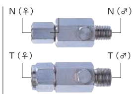
逆止弁 (チェックバルブ) ■Nタイプ (上) 税込価格 ¥15,400 ■Tタイプ (下) 税込価格 ¥15,400 ※エアの流れを一方にしか流さないようにする金具です。革パッキン1枚付。
