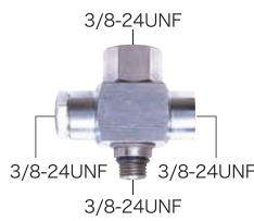
3ポート低圧アダプター (LPプラグ1個付)
