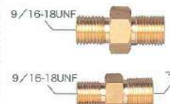
異径ジョイント金具(異径ニップル)
