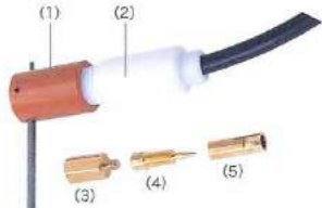
水中溶接(切断)用ホルダーセット
