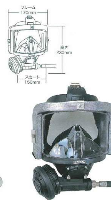
アガマスクセット ブラックシリコン
