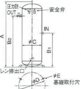
貯気空気タンク
