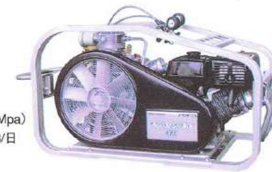
ユーティラス(モーター) (充填)23分(12ℓ・19.6Mpa) エア噴出量:144m3/日 サイズ:L90×W40×H50cm モーター付:71kg エンジン付:73kg
