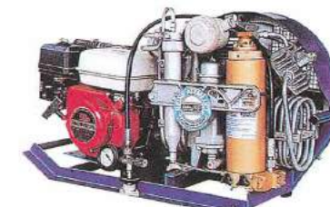
キャピタノ(ディーゼル) (充填)15分(12ℓ・19.6Mpa) エア噴出量:201.6m3/日 サイズ:L90×W40×H50cm モーター付:77kg エンジン付:79kg ディーゼル付:117kg
