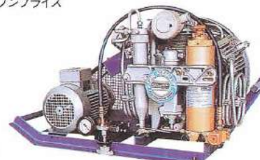
ユーティラス(モーター) (充填)23分(12ℓ・19.6Mpa) エア噴出量:144m3/日 サイズ:L90×W40×H50cm モーター付:71kg エンジン付:73kg
