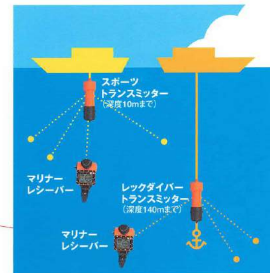
ES-203 TXレックダイバートランスミッター (送信機)
