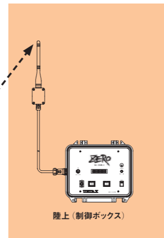
無線通信制御
