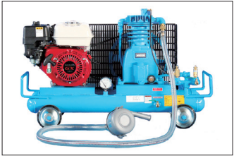
GE-15E-13 (改) 〈低圧型エンジン駆動〉
