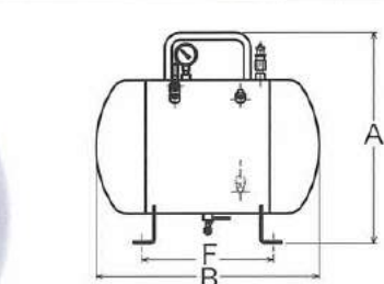
貯気空気タンク
