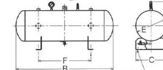
貯気空気タンク(横型)
